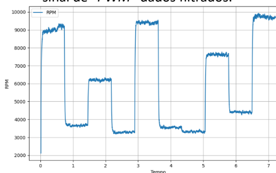
Figura 7 - Resposta no tempo do cooler ao sinal de “PWM” dados filtrados.
